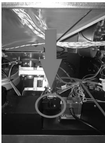
Fig. 42 - Manueller Reset: Befindet sich hinter dem Tank in der Nähe des Versorgungssteckers
