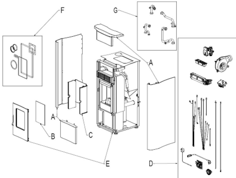
Fig. 1 - Explosionszeichnung
