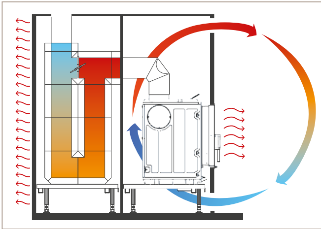
Abb. 10: Heizkreislauf, Schema
