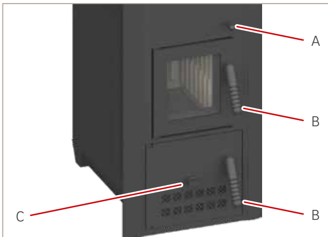
Abb. 18: Bedienelemente am Beispiel Creation 6
