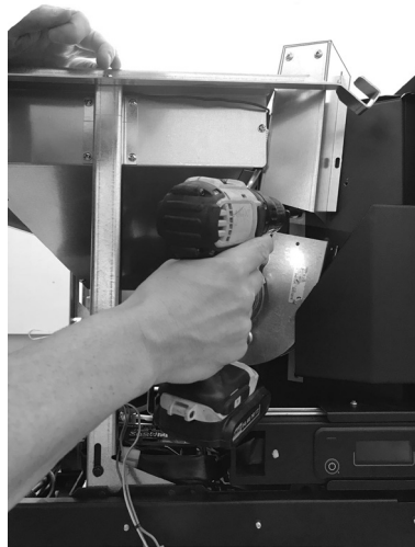
Fig. 45 - Gebläse befestigen
