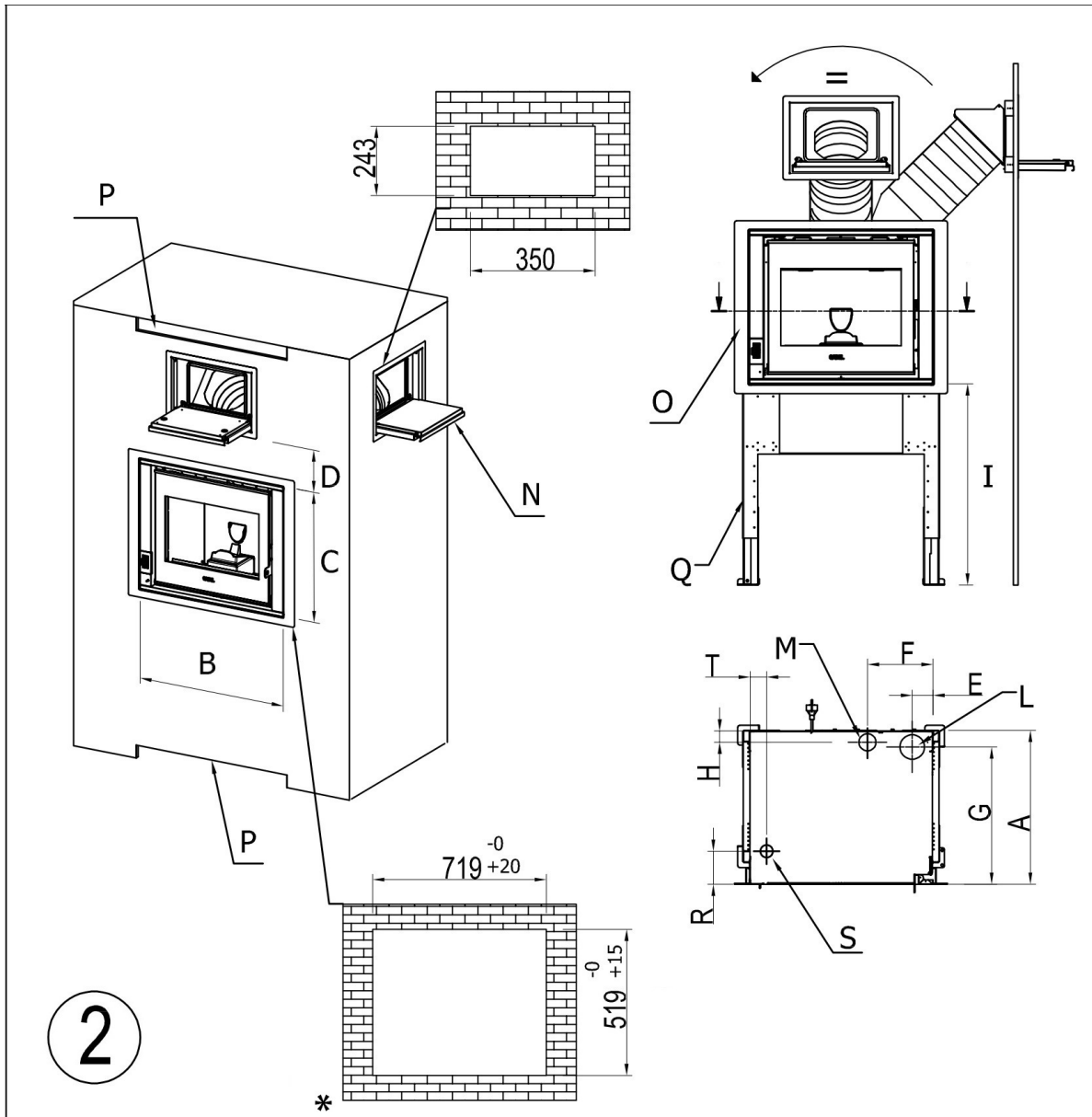
Fig. 15 - ZEN ZEFIRO mit Falltür + Rahmen
