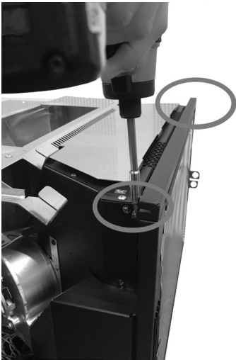
Fig. 51 - Oberes Profil entfernen
