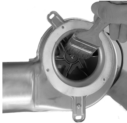
Fig. 99 - Reinigung 2
