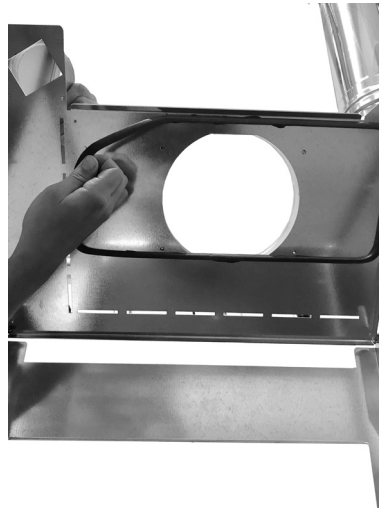
Fig. 52 - Dichtung entfernen
