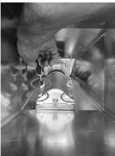
Fig. 89 - Lösen der Schrauben
