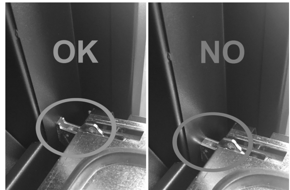
Fig. 71 - Korrektes Ankuppeln des Scharniers
