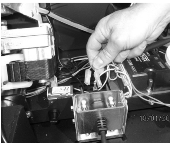
Fig. 86 - Trennen Faston-Stecker (blau - braun)
