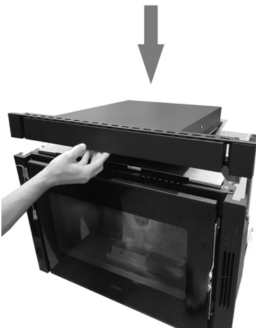
Fig. 54 - Schublade positionieren
