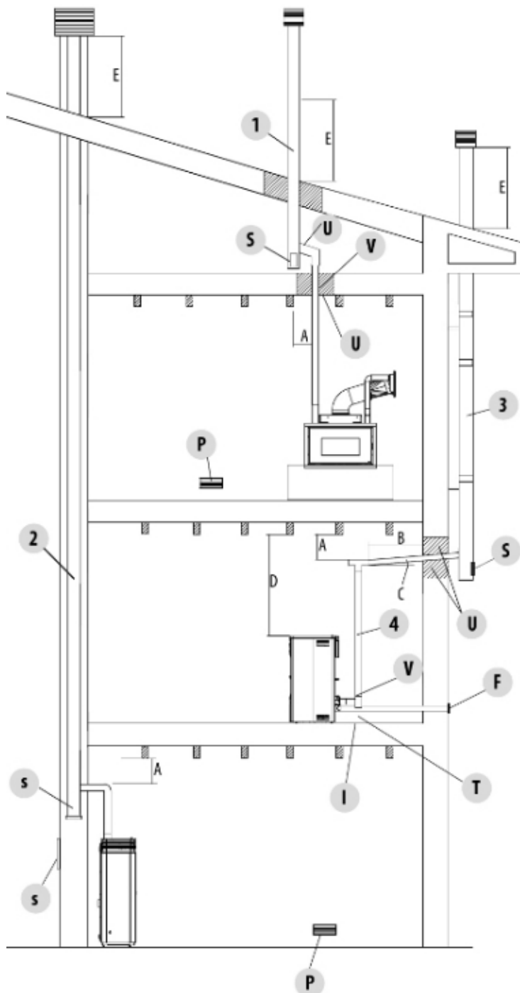
Fig. 12 - Rauchabzug
