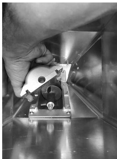
Fig. 90 - Gehäuse entfernen
