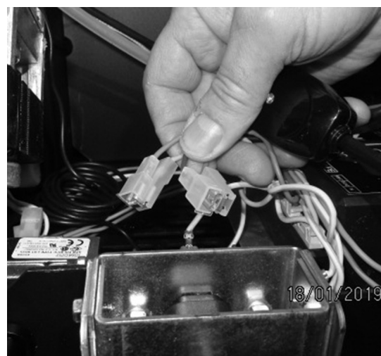
Fig. 87 - Anschluss Doppel-Faston-Buchsen
