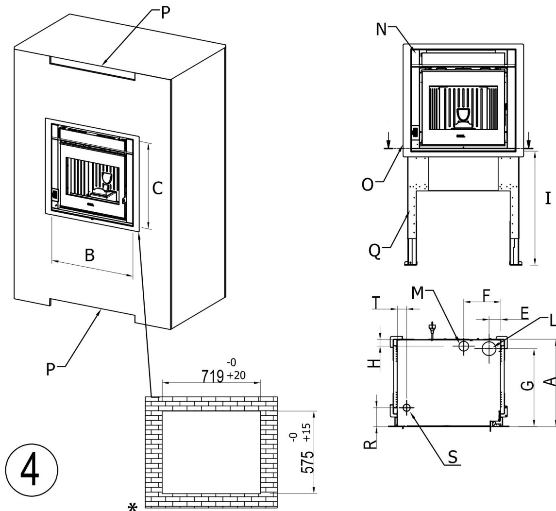
Fig. 17 - ZEFIRO-ZEN Lade+ Rahmen
