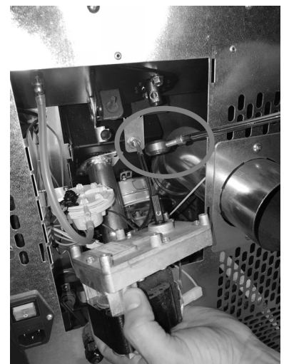
Fig. 91 - Getriebemotor entfernen
